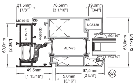
Porte Terrasse avec Périmètre de 114,3mm (4 1/2") Terrace Door with 114,3mm (4 1/2") Perimeter Frame
