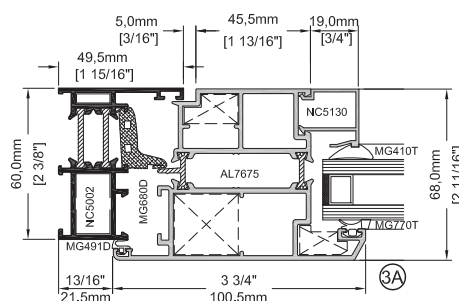
Porte Terrasse avec Périmètre de 114,3mm (4 1/2") Terrace Door with 114,3mm (4 1/2") Perimeter Frame
