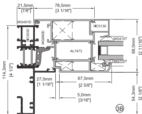
Porte Terrasse avec Périmètre de 114,3mm (4 1/2") Terrace Door with 114,3mm (4 1/2") Perimeter Frame
