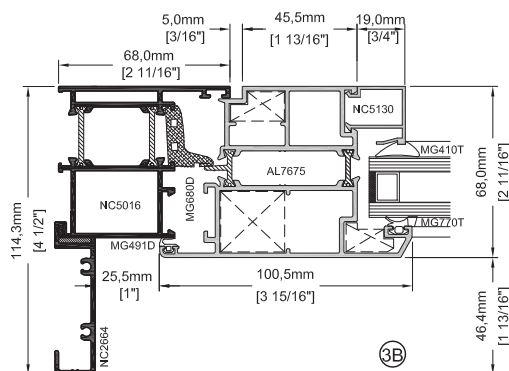
Porte Terrasse avec Périmètre de 114,3mm (4 1/2") Terrace Door with 114,3mm (4 1/2") Perimeter Frame
