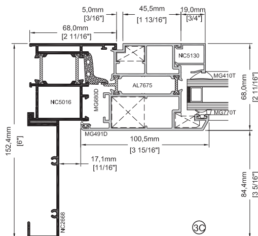
Porte Terrasse avec Périmètre de 152,4mm (6") Terrace Door with 152,4mm (6") Perimeter Frame
