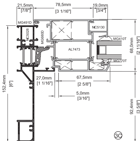
Porte Terrasse avec Périmètre de 152,4mm (6") Terrace Door with 152,4mm (6") Perimeter Frame
