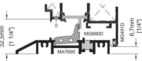
Seui ADA en Option ADA Threshold in Option
