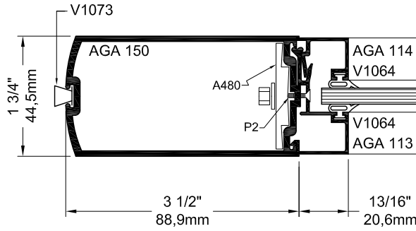
Battant de rencontre Meeting stile
