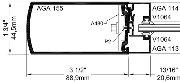
Battant de rencontre Meeting stile
