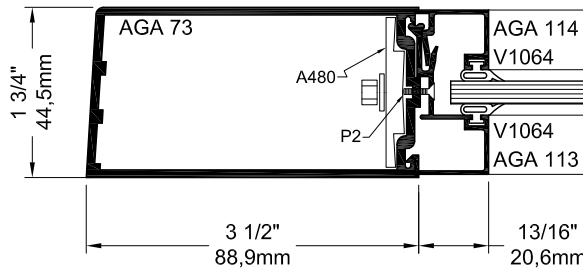
Battant décentré Offset stile
